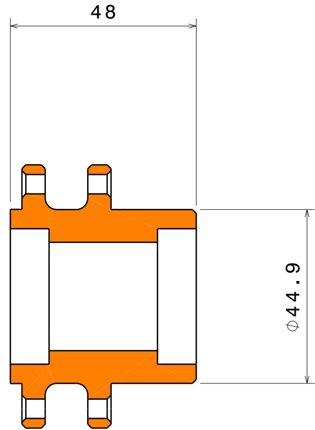
Section view A-A Scale: 1:1
